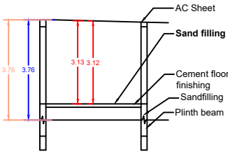
SECTION - AB
