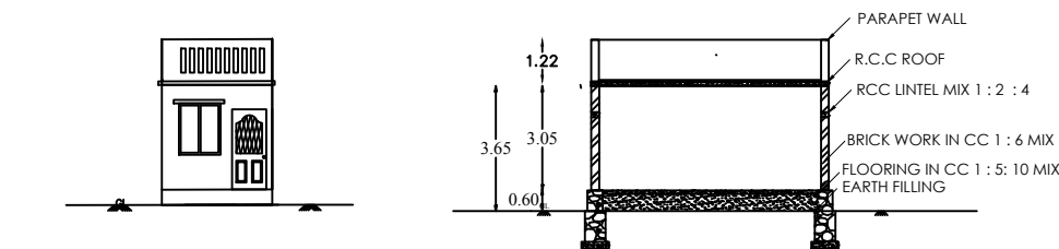
ELEVATION
