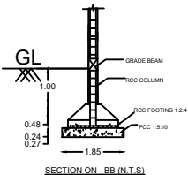
SECTION ON - BB (N.T.S)
