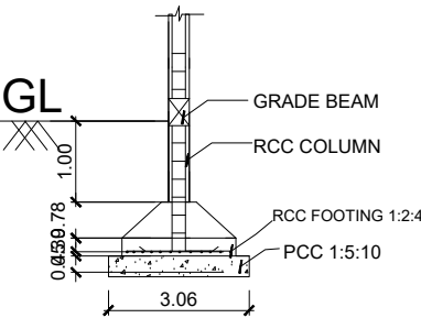
SECTION ON - BB (N.T.S)
