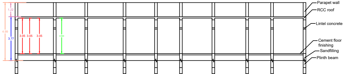
SECTION - AB
