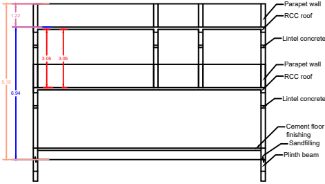
SECTION - AB
