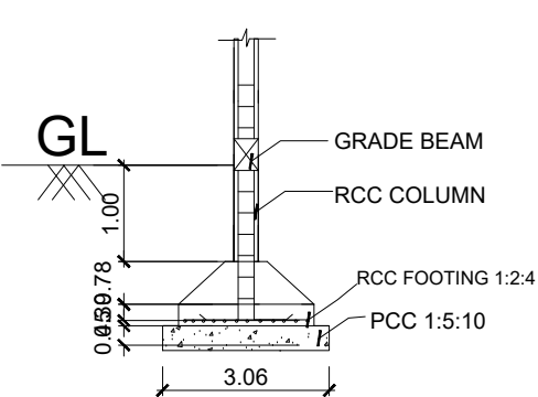
SECTION ON - BB (N.T.S)
