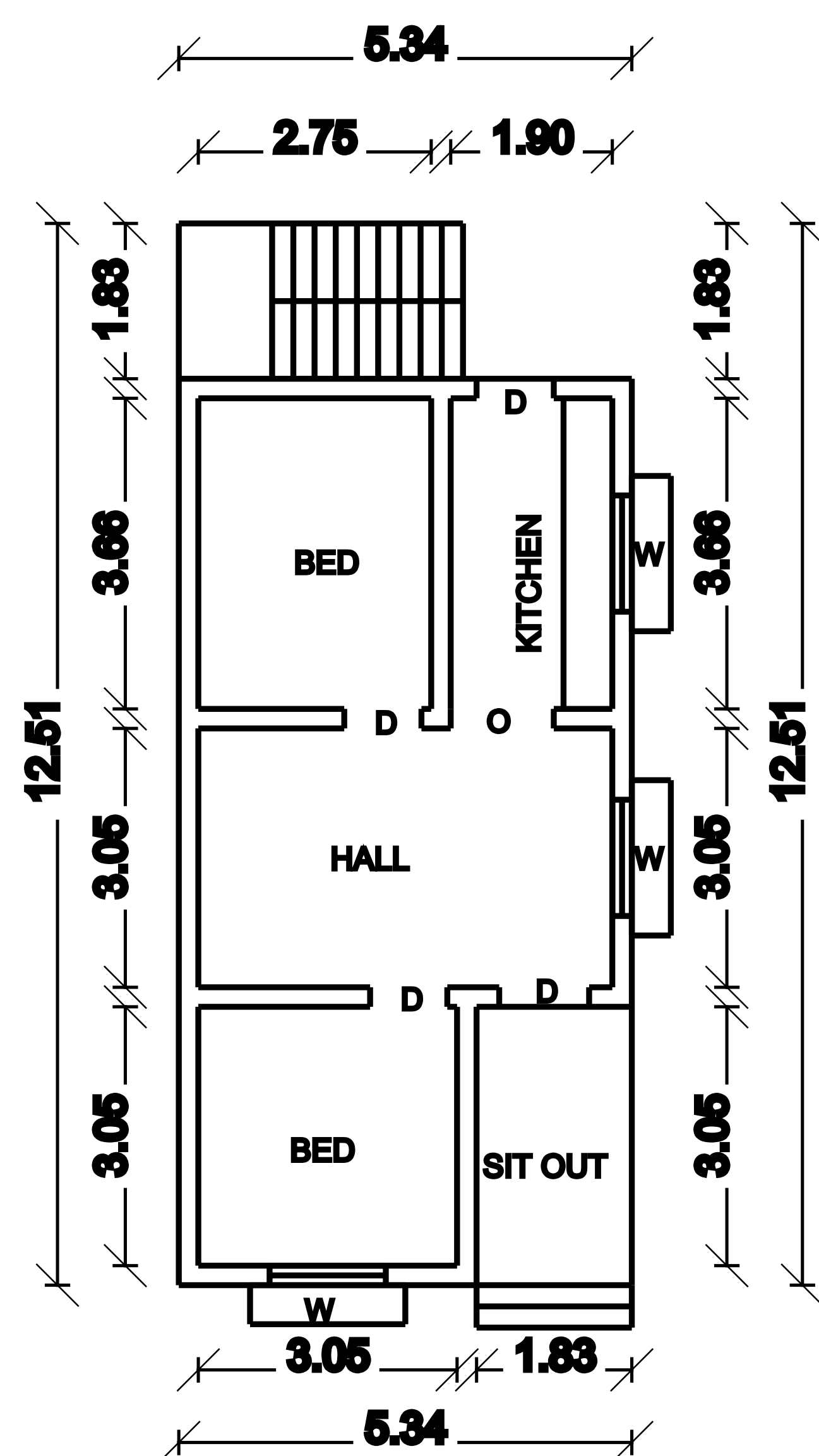
G.F PLAN
