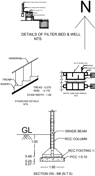
SECTION ON - BB (N.T.S)
