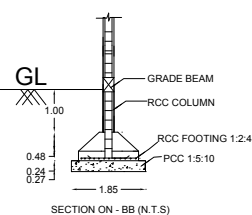
SECTION ON - BB (N.T.S)
