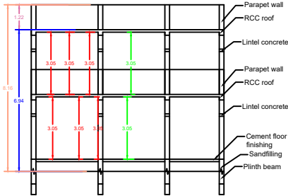
SECTION - AB
