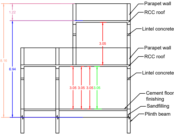
SECTION - AB
