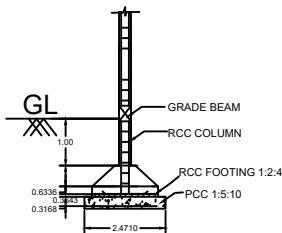
SECTION ON - BB (N.T.S.)
