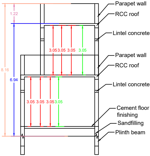
SECTION - AB
