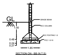
SECTION ON - BB (N.T.S)
