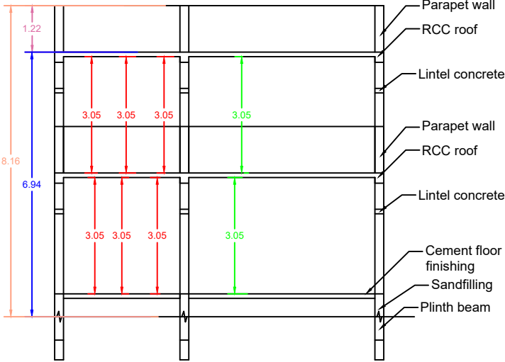
SECTION - AB
