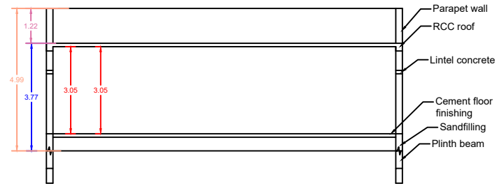
SECTION - AB
