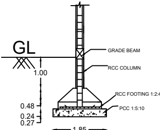
SECTION ON - BB (N.T.S.)
