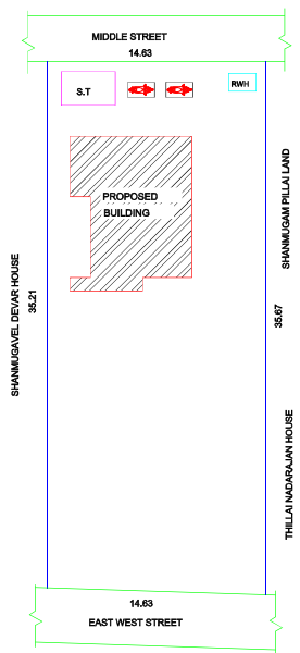
SITE PLAN (SCALE 1:200)
