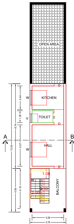
F.F. PLAN
