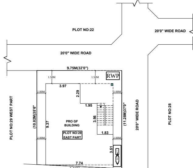
S.NO: 6/ 2 LAND SITE PLAN SCALE 1:100
