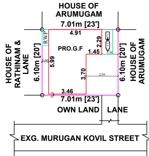
SITE PLAN SCALE 1:100
