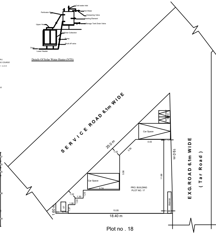
SITEPLAN
