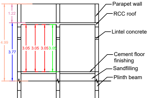
SECTION - AB
