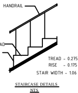
NTS
