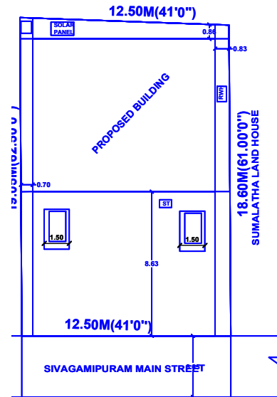
SITE PLAN SCLAE 1CM:1METER
