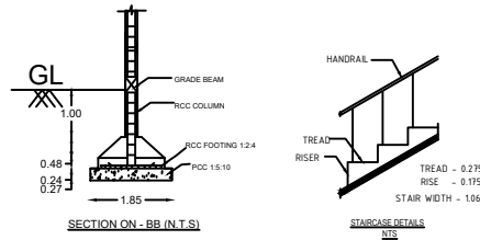
SECTION ON - BB (N.T.S)
