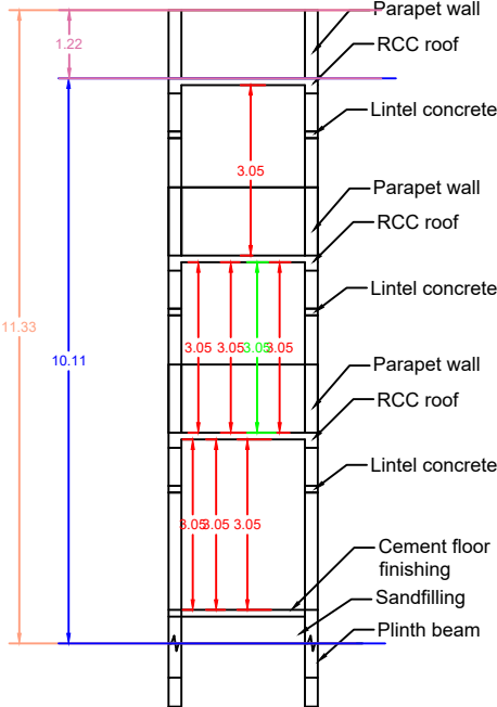
SECTION - AB
