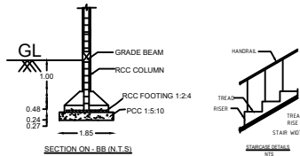
SECTION ON - BB (N.T.S.)
