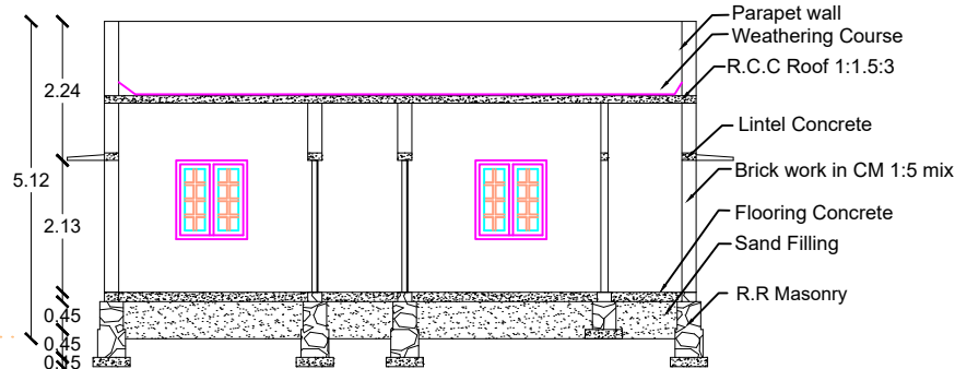
SECTION-E1E1
