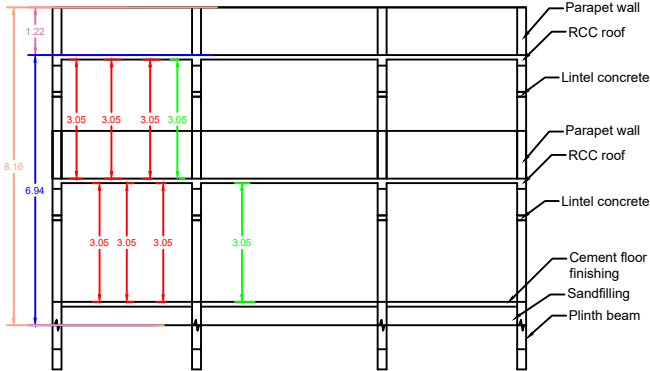
SECTION - AB
