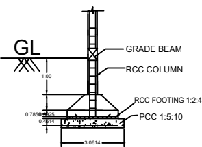
SECTION ON - BB (N.T.S)
