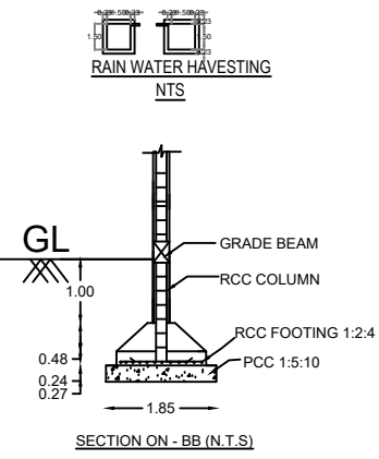
SECTION ON - BB (N.T.S)
