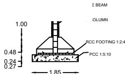
SECTION ON - BB (N.T.S)
