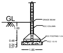
SECTION ON - BB (N.T.S)
