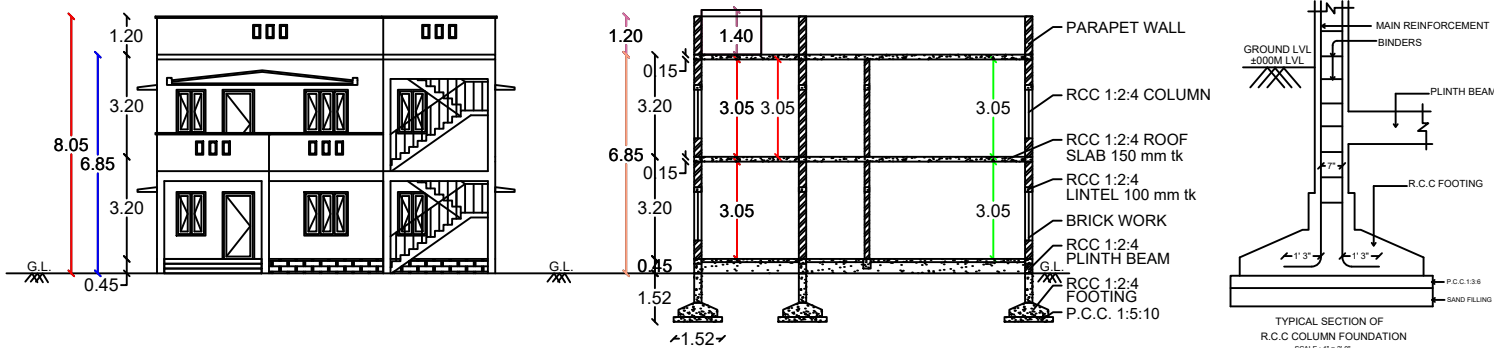
ELEVATION
