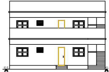
ELEVATION
