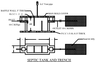
SECTION - AB
