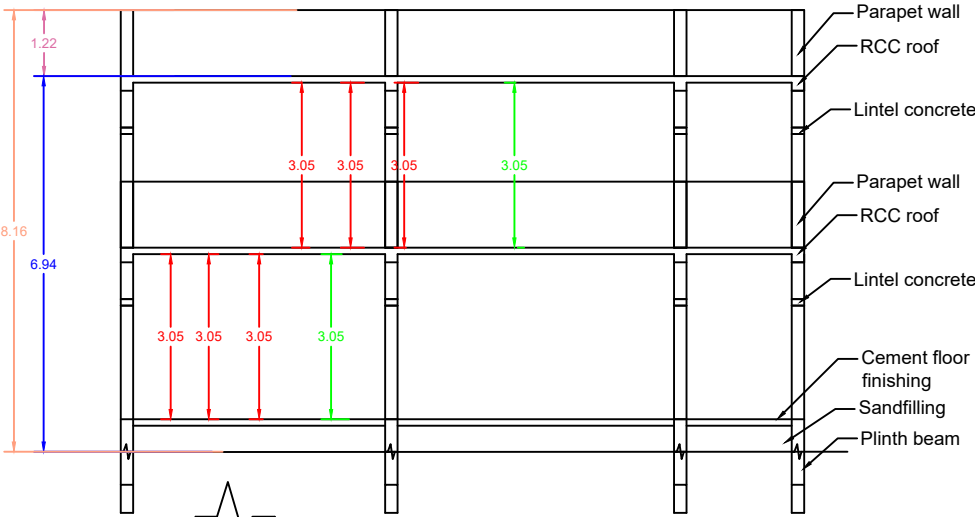
SECTION - AB
