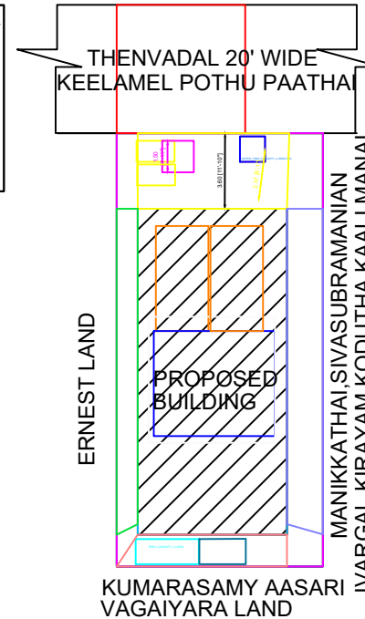
SITE PLAN(SCALE 1:100)
