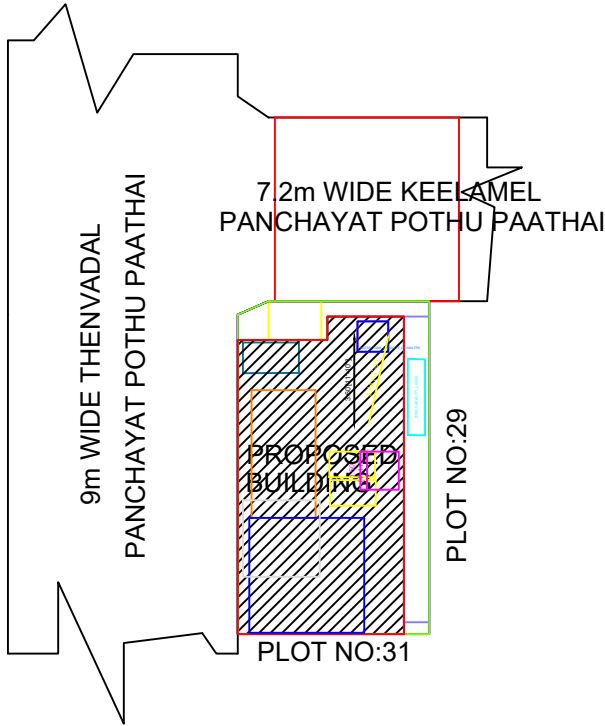
SITE PLAN(SCALE 1:100)
