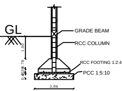
SECTION ON - BB (N.T.S)
