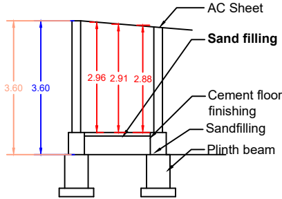
SECTION - AB
