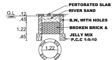
R.W.C.T, PLAN & SECTION
