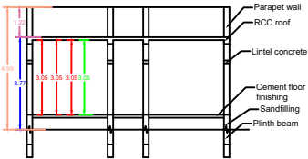
SECTION - AB
