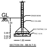
SECTION ON - BB (N.T.S.)
