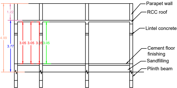
SECTION - AB
