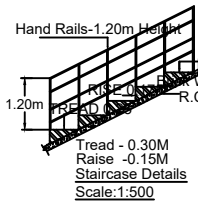
Scale:1:500
