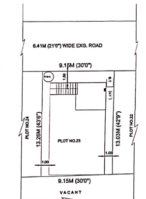
SITE PLAN 1:200
