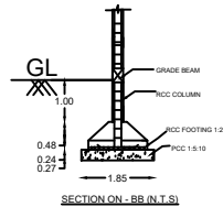
SECTION ON - BB (N.T.S)
